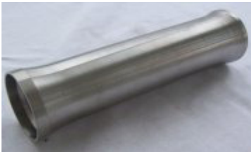
Steuerrohr Dedacciai f. Campa Integrated Headset 165mm Aussendurchmesser im Mittelteil 39.5mm (Fräswerkzeug dazu kann geliehen werden)
